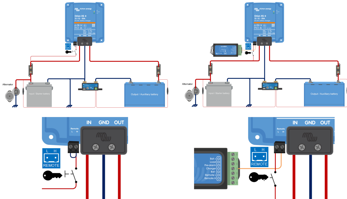
Diagrama de ligação da anulação da detecção de motor desligado
